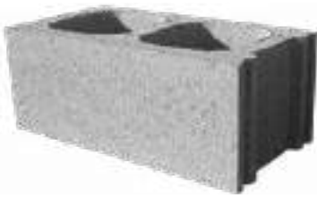
BLOCCO 25 - 25X20X50
