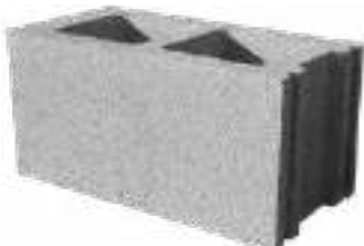
BLOCCO 2050 - 20X20X50
